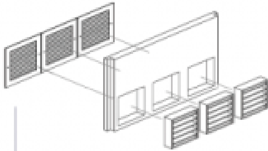
ENSAMBLE VENTILACIONES 150x150
